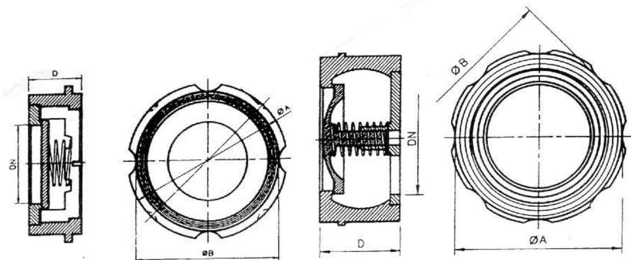
Type 048050/70/80, DN 15 – 100
