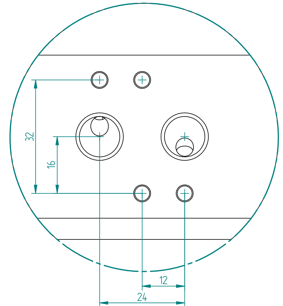
DETAIL A 1,5:1
