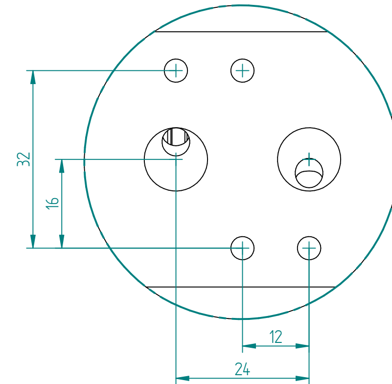
DETAIL A 1,5:1
