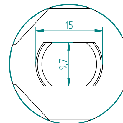
DETAIL A 2:1
