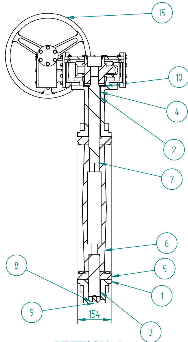
SECTION A-A
