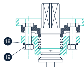
A-A VIEW
