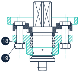
A-A VIEW
